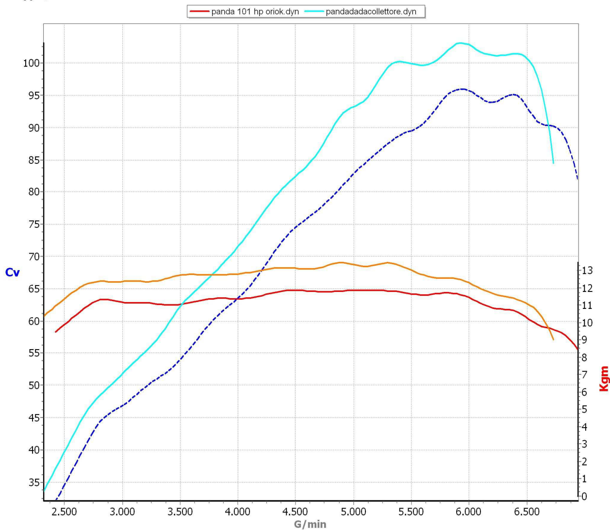
Coppia/Potenza Motore
